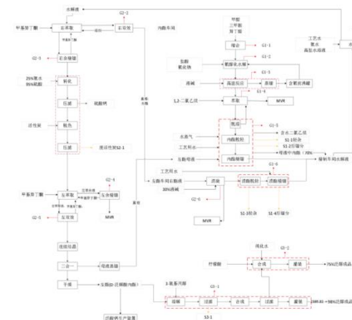
新酯项目生产工艺流程图
